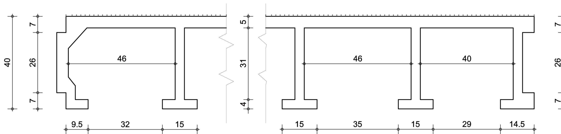
DEKDEELPROFIEL (schaal 1:1)
